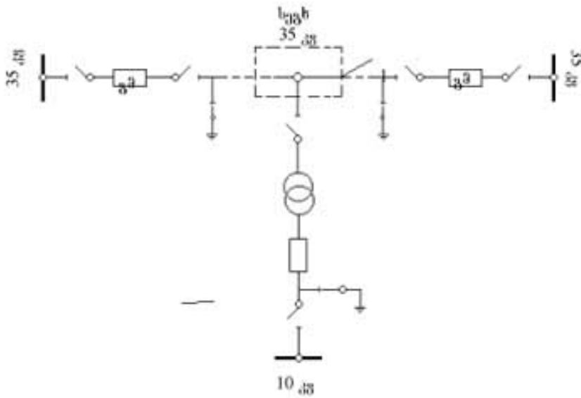
დანიშნულება 6.1. 35 კვ საბაჟური ხაზზე (განმარტობაზე ქვესადგურით) დამსწების დაცვების მაგალითი წინამდებარე წესების 3.6.1. პუნქტის მიხედვით (დამსწების საბაჟური ადგილიზე ნაჩვენებია არ არის); 1 – საბაჟური ადგილი (საბაჟური უბანი)
